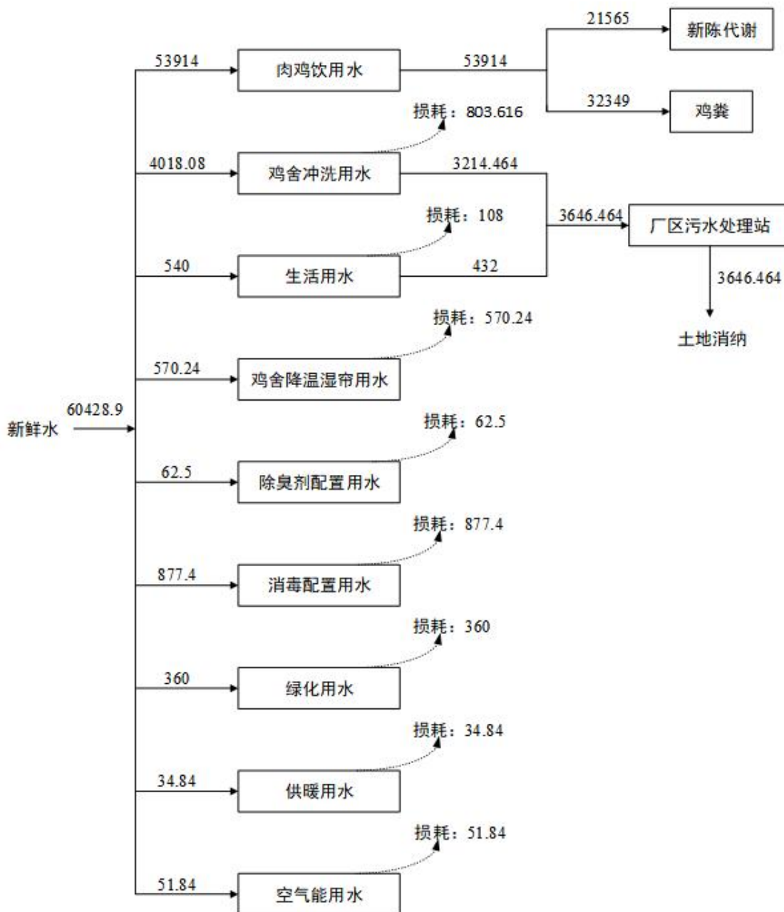
图 3.4-1 项目水平衡 (m³/a)
